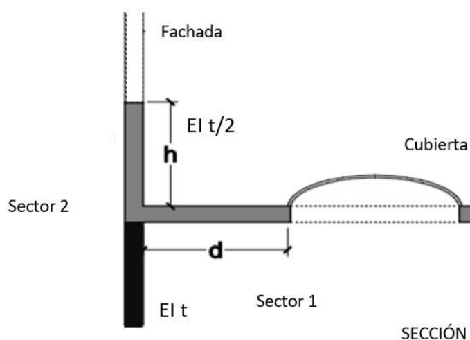
Figura 2.15: Encuentro cubierta-fachada
