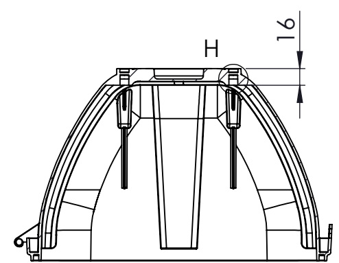
DETALLE G
